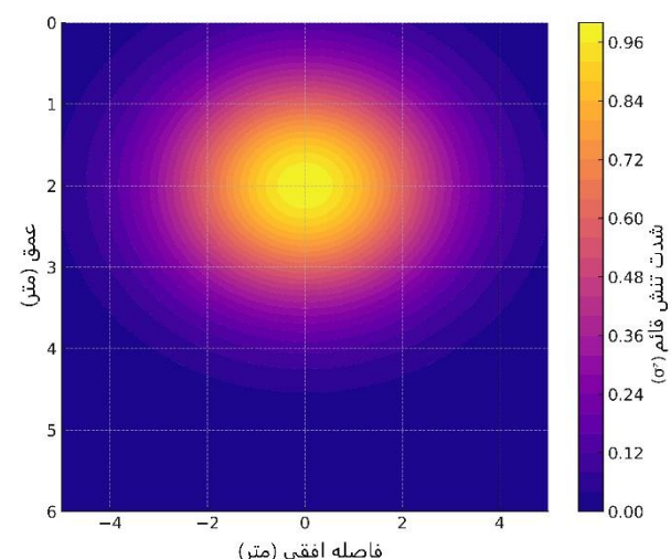
شکل ۲ - توزیع تنش قائم در مدل عددی ستون سنگی تزریق‌شده
